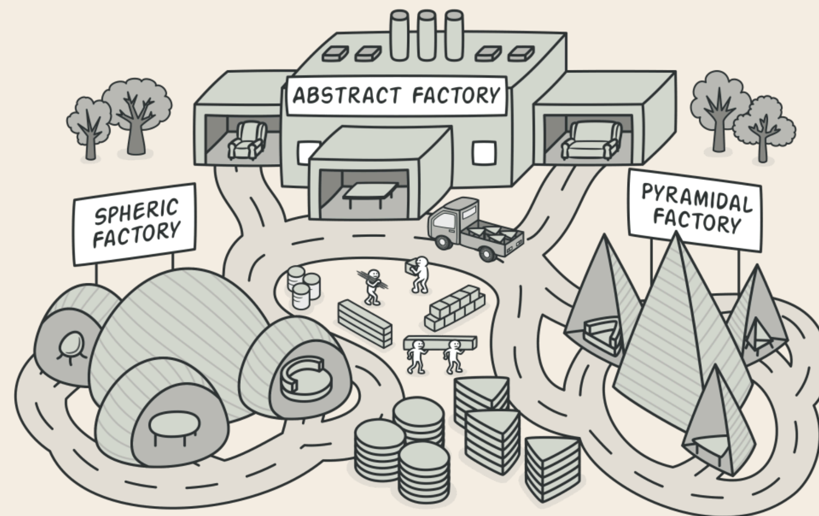
Hình ảnh minh họa khái niệm Xưởng trừu tượng bởi Refactoring.Guru
