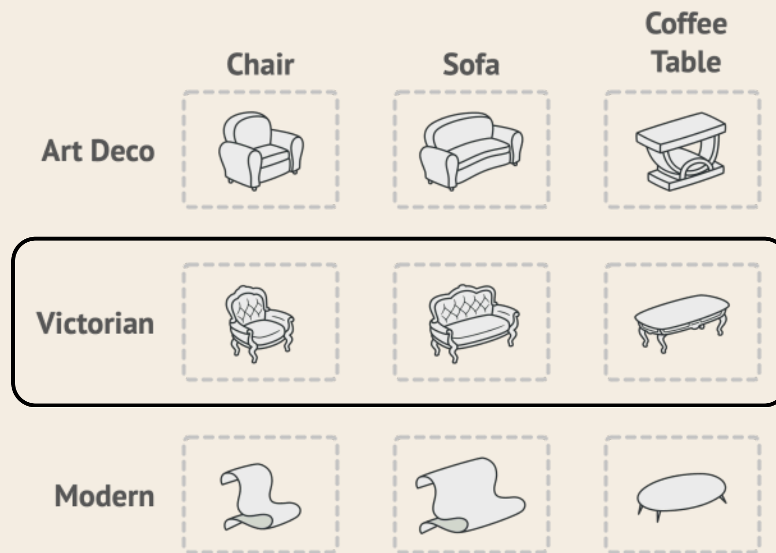
Hình ảnh minh họa các đối tượng cần định nghĩa bởi Refactoring.Guru
