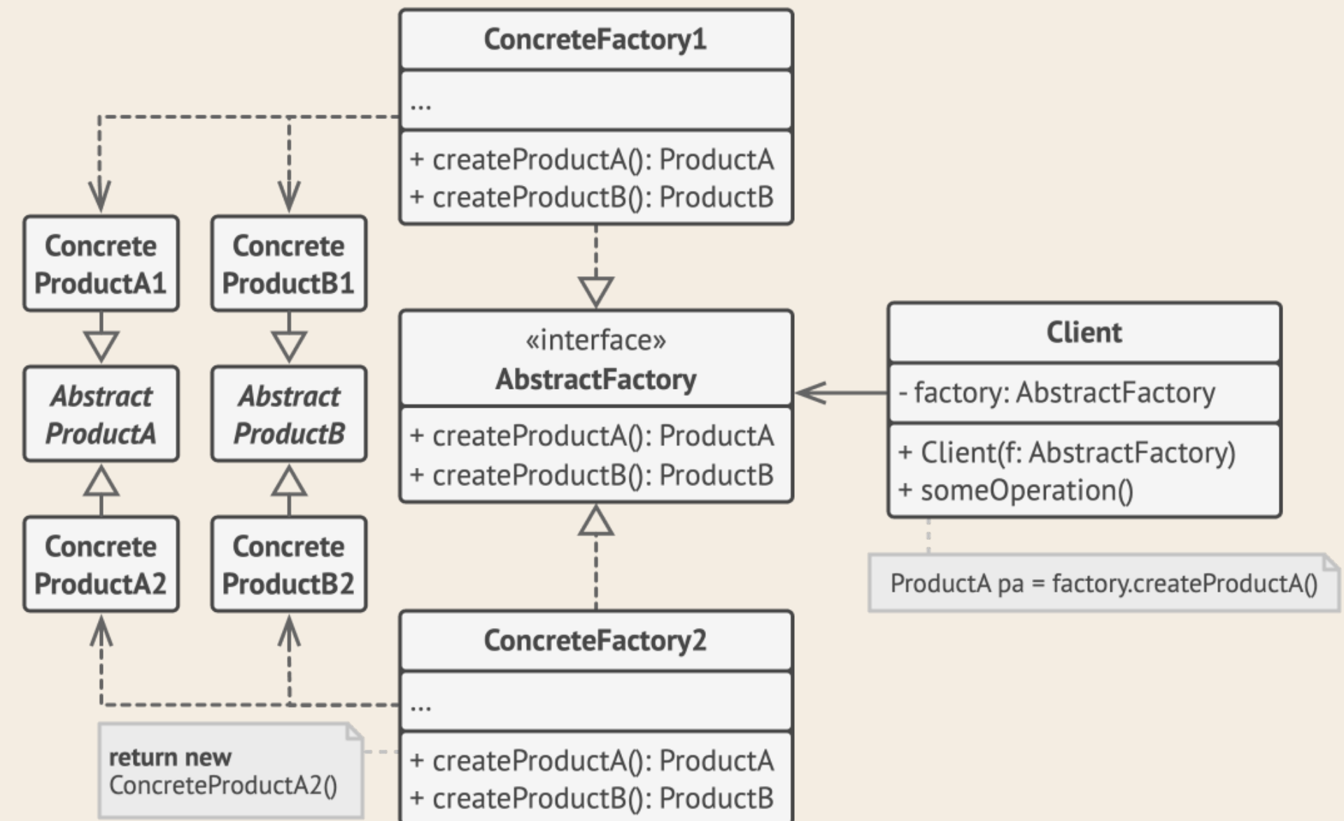
Hình ảnh minh họa cấu trúc mẫu thiếu kế xưởng trừu tượng bởi Refactoring.Guru
